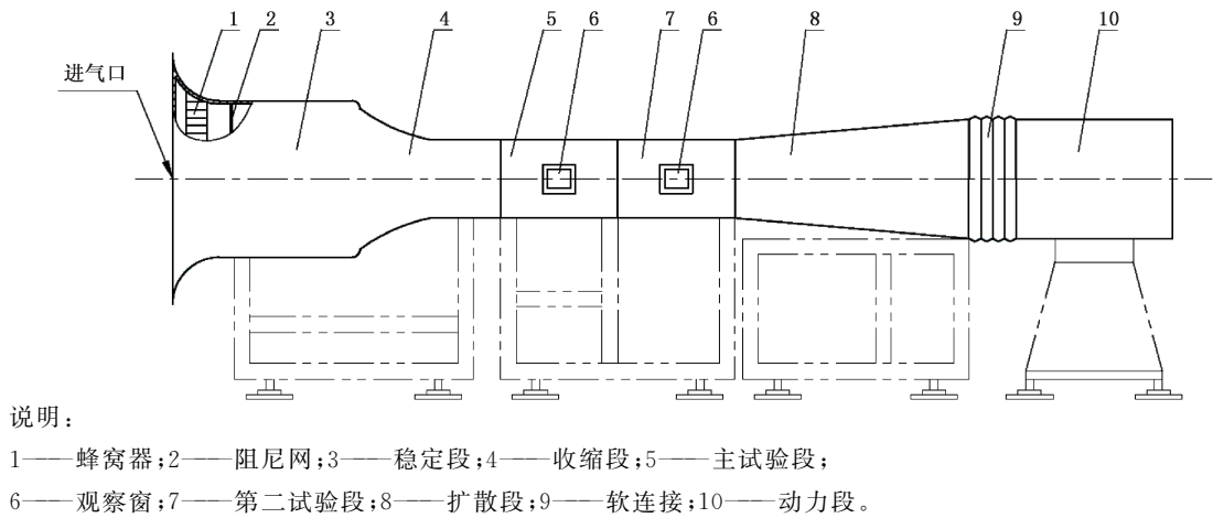
图 1 直流式风洞示意图
