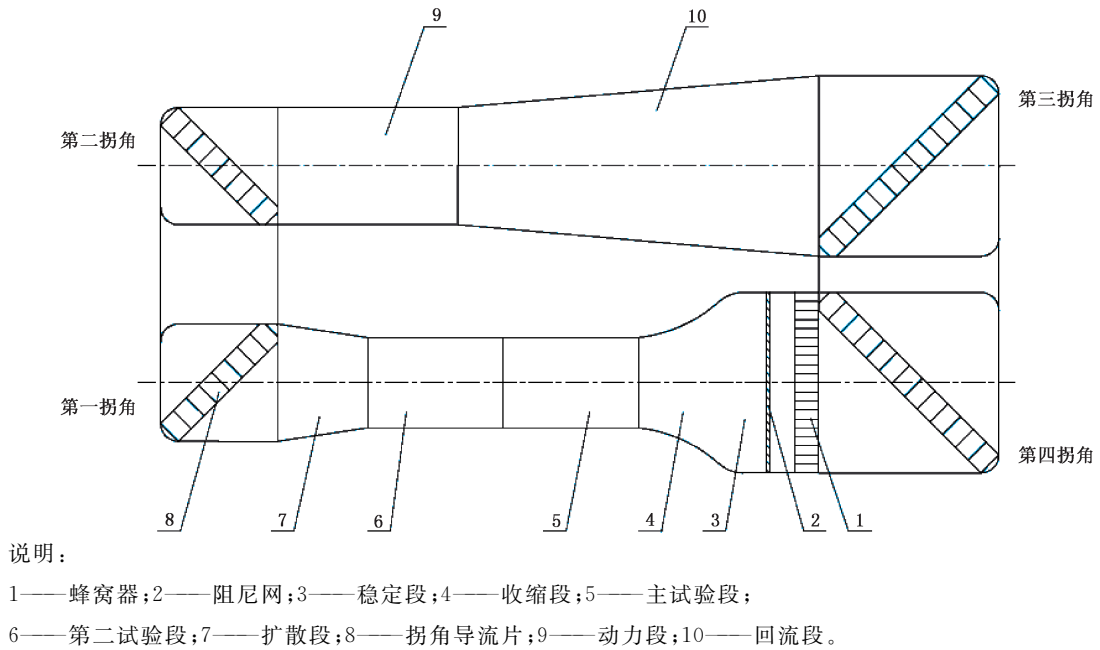
图 2 单回流式风洞鸟瞰示意图
